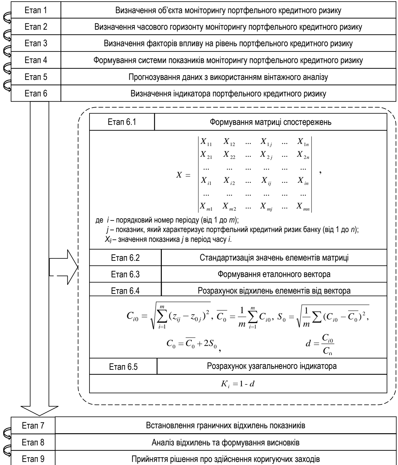
Рисунок 5 – Загальний алгоритм визначення індикатора портфельного кредитного ризику та його моніторингу
